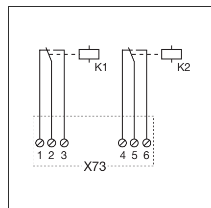
7-2.3 Schaltplan der Relais
