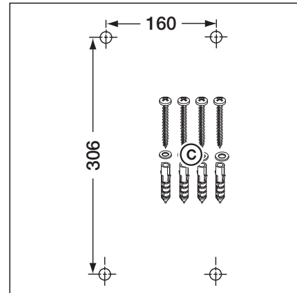
3-2.6 Bohrbild der Befestigungslöcher, benötigtes Montagmaterial
