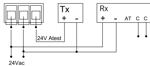
LICHTSCHRÄNKE OHNE AUTOTESTANSCHLUSS
