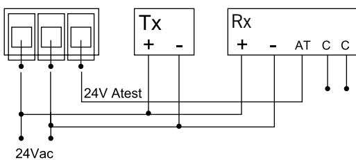
LICHTSCHRÄNKE MIT AUTOTESTANSCHLUSS
