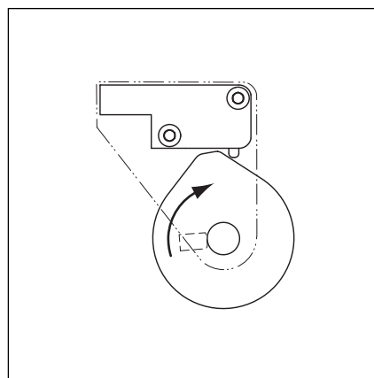
6-14.5 Schaltrichtung des Schaltnockens S2 - Sicherheits-Endschalter Tor-Zu -
