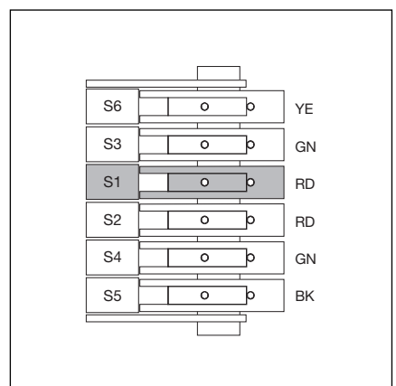
6-13.4 Schalnocke S1 - Sicherheits-Endschalter Tor-Auf -
