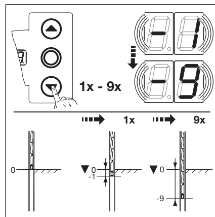
6-9.2 Endlage Tor-Zu weiter Richtung Tor-Zu einstellen
