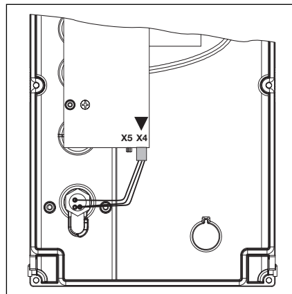
6-26.1 Anschluss des Miniaturschlusses, Deckelinnenseite, von X5 nach X4 umstecken.
