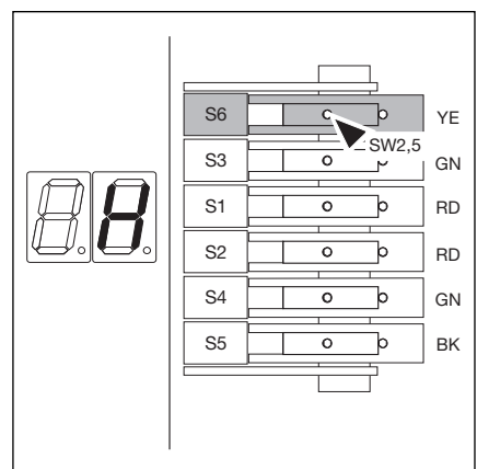
6-18.4 Anzeige Zwischenendlage, Nocken festsetzen
