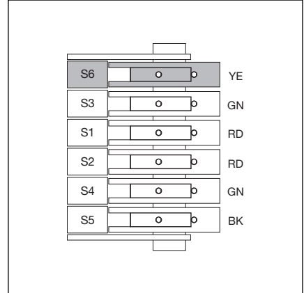
6-18.2 Schaltknocke S6 - Zwischenendlage (1/2-Auf) -
