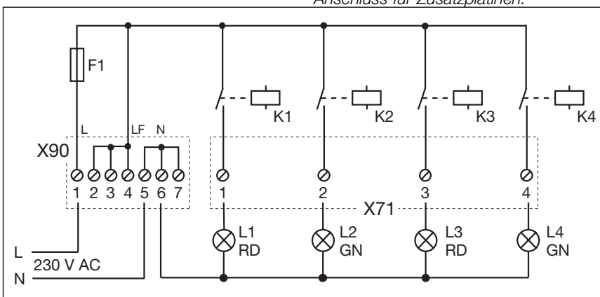
7-4.4 Schaltplan Stromversorgung und Relais
