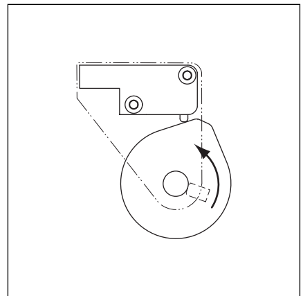
6-13.2 Schaltrichtung des Schalnockens S3 - Endlage Tor-Auf -
