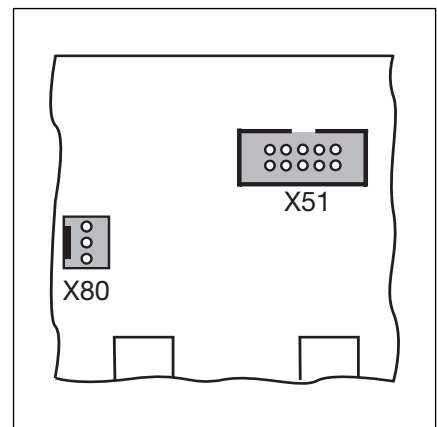
7-8.2 X51 = Anschluss zur Steuerung, X80 = Anschluss für Zusatzplatinen.
