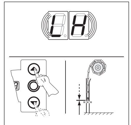
6-11.1 Zwischenendlage Tor-Auf einlernen
