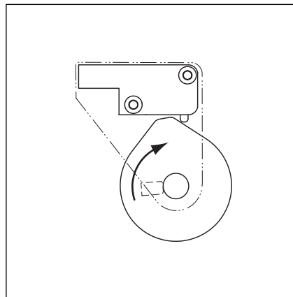
6-15.3 Schaltrichtung des Schaltnockens S5 - SKS-Stopp -
