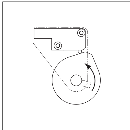
6-13.5 Schaltrichtung des Schalnockens S1 - Sicherheits-Endschalter Tor-Auf -
