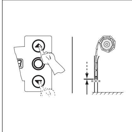
6-18.1 Position Zwischenendlage anfahren
