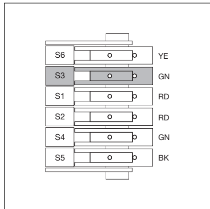
6-13.1 Schalnocke S3 - Endlage Tor-Auf -
