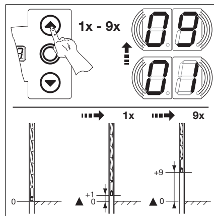
6-9.1 Endlage Tor-Zu zurück Richtung Tor-Auf einstellen
