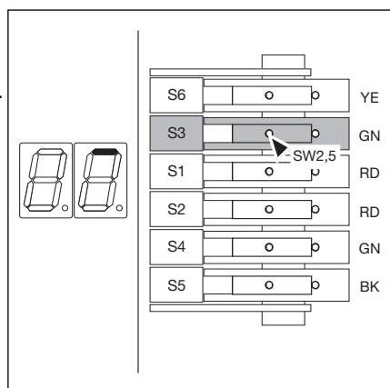
6-13.3 Anzeige Endlage Tor-Auf, Nocken festsetzen
