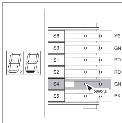
6-14.3 Anzeige Endlage Tor-Zu, Nocken festsetzen
