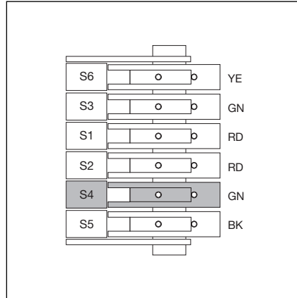
6-14.1 Schaltnocke S4 - Endlage Tor-Zu -
