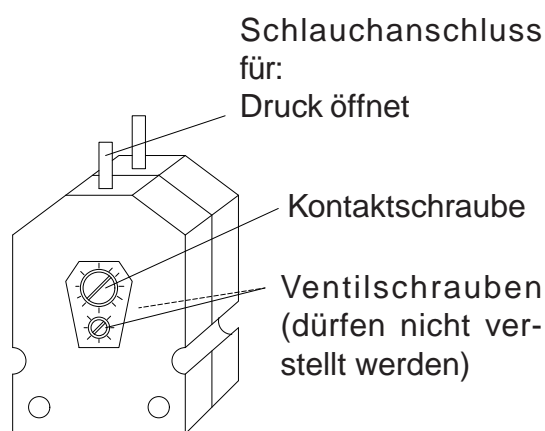
Druckwellenschalter
