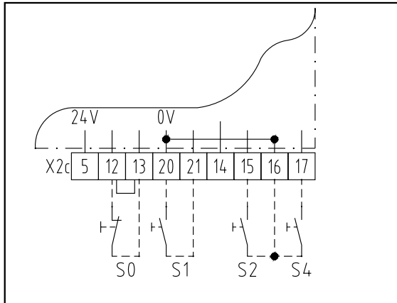
Abb. 15: Schaltplan
