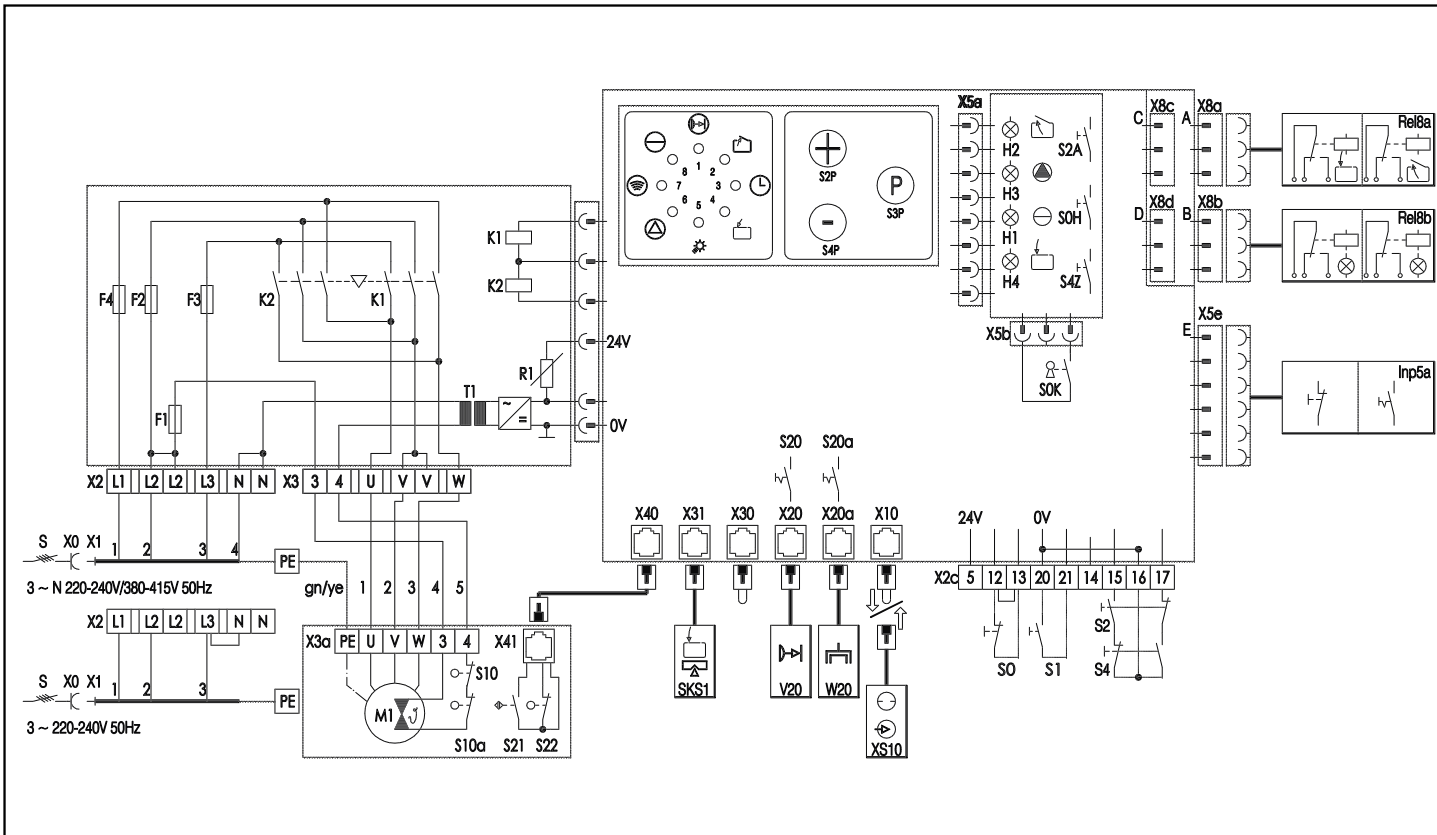
Abb. 25: Schaltplan
