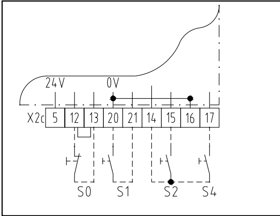
Abb. 17: Schaltplan
