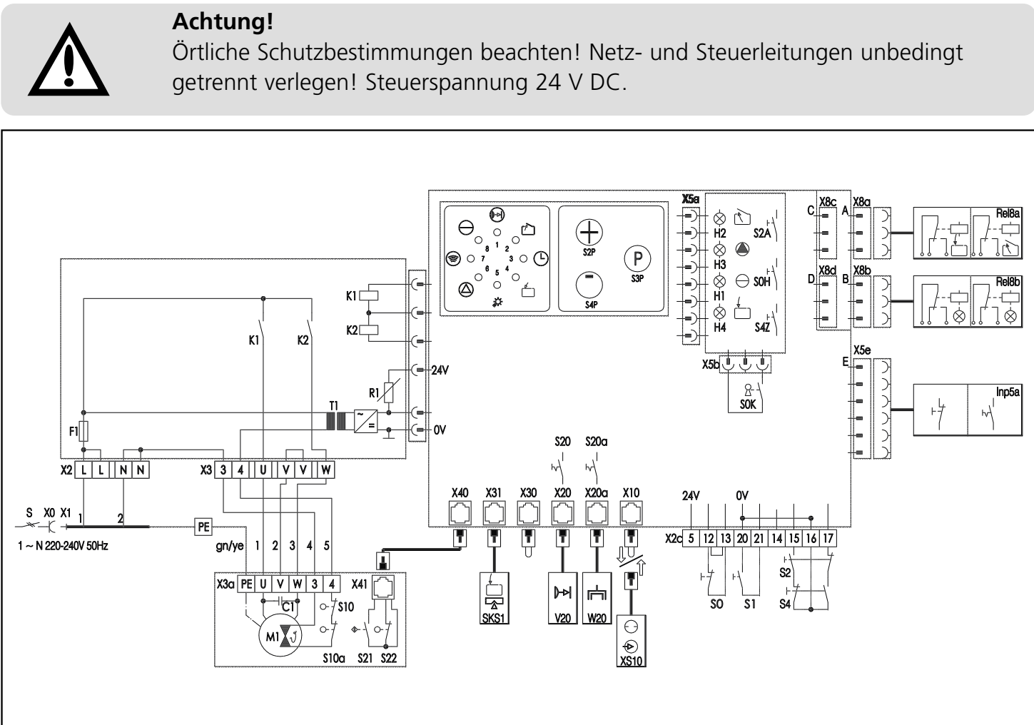
Abb. 26: Schaltplan
