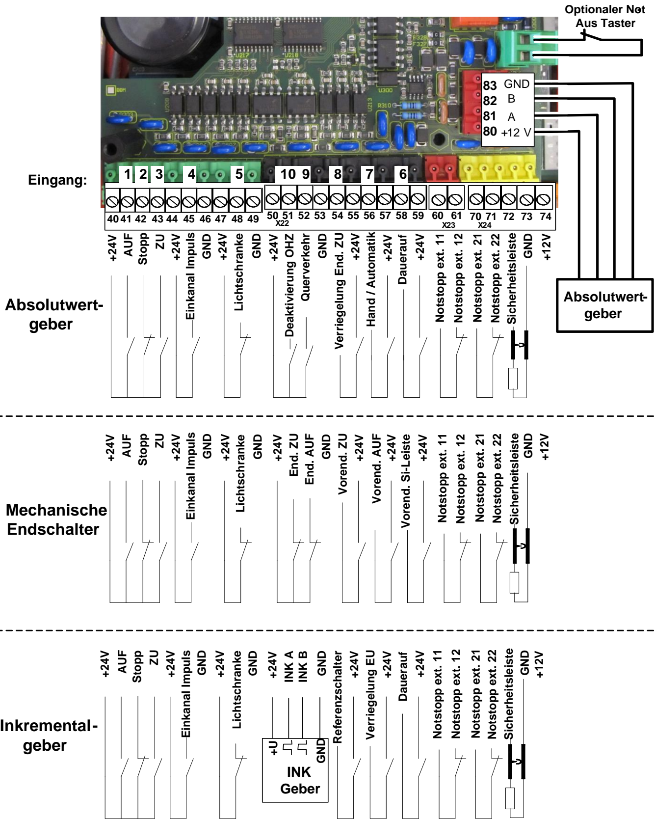
Abbildung 18: Eingänge
