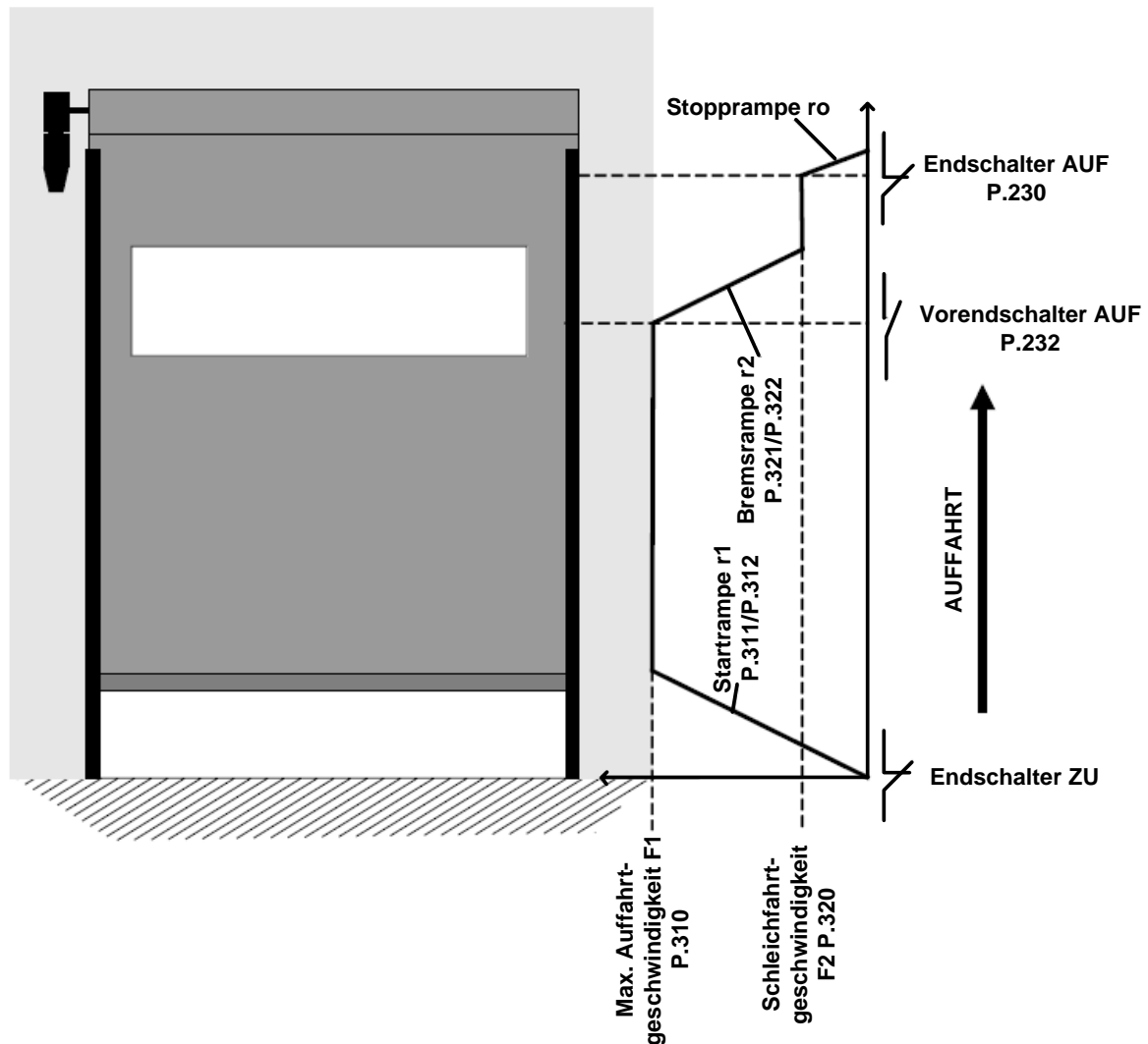
Abbildung 23: Auffahrt mit Frequenzumrichter
