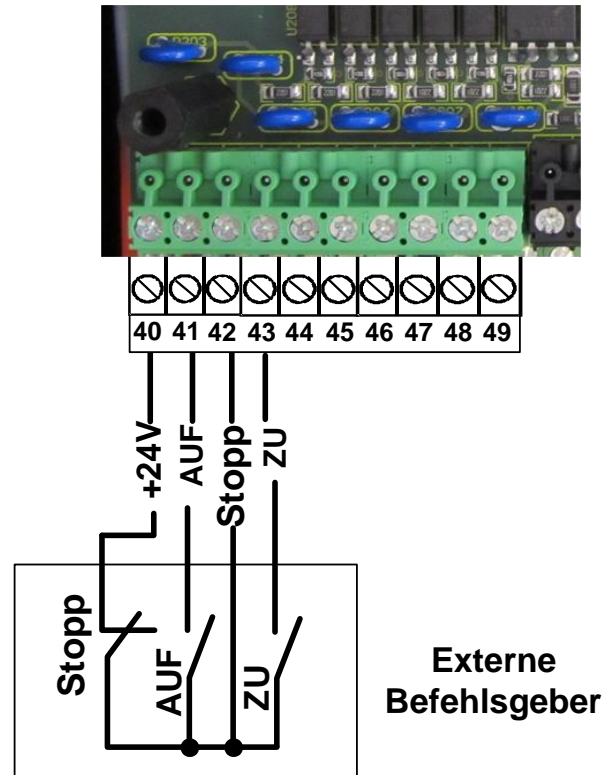
Abbildung 16: Anschluss externe Befehlsgeber
