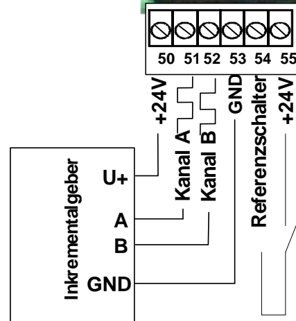
Abbildung 14 Anschluss Inkrementalgeber
