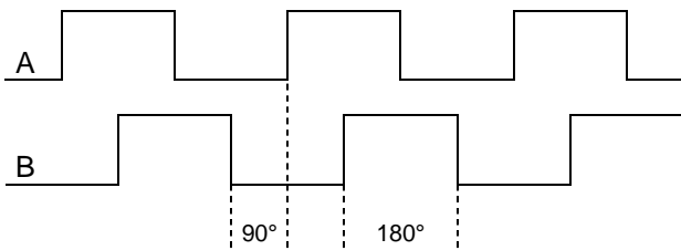
Abbildung 13: Funktionsweise Inkrementalgeber
