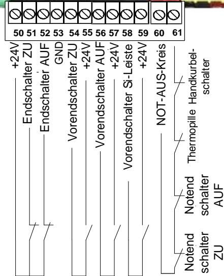
Abbildung 11: Anschluss Nockenendschalter
