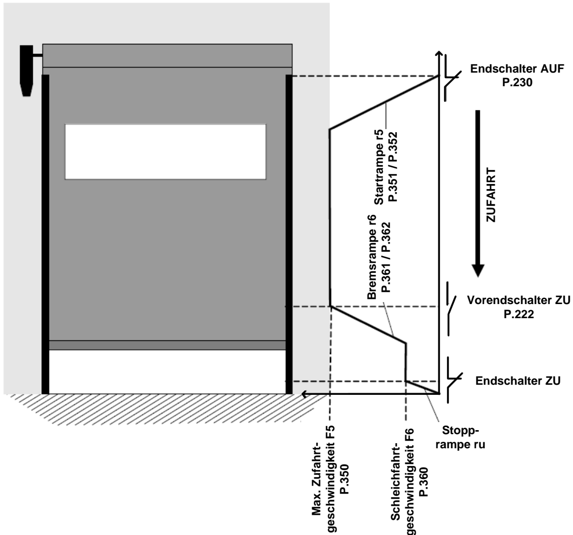
Abbildung 24: Zufahrt mit Frequenzumrichter
