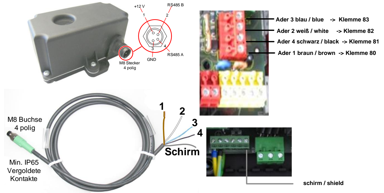
Abbildung 8: Anschluss des Absolutwertgeber TST PD
