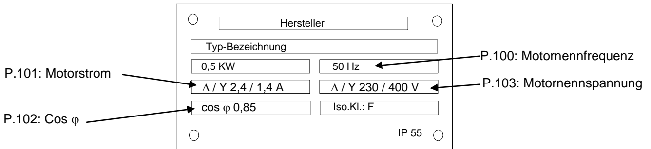
Abbildung 21: Beispiel Motortypenschild (Abb. ähnlich)
