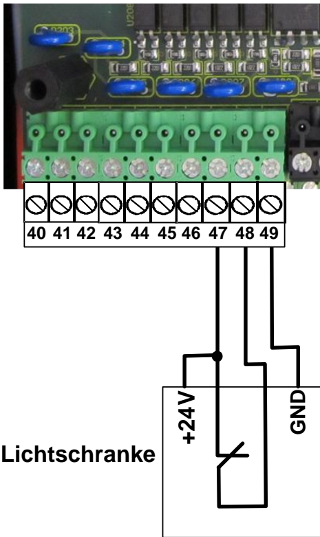
Abbildung 15: Anschluss Lichtschanke
