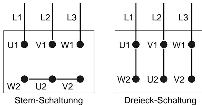
Abbildung 22: Stern- / Dreieckschaltung
