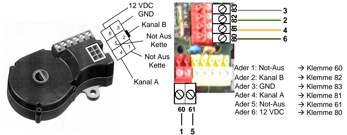
Abbildung 9: Anschluss Absolutwertgeber DES
