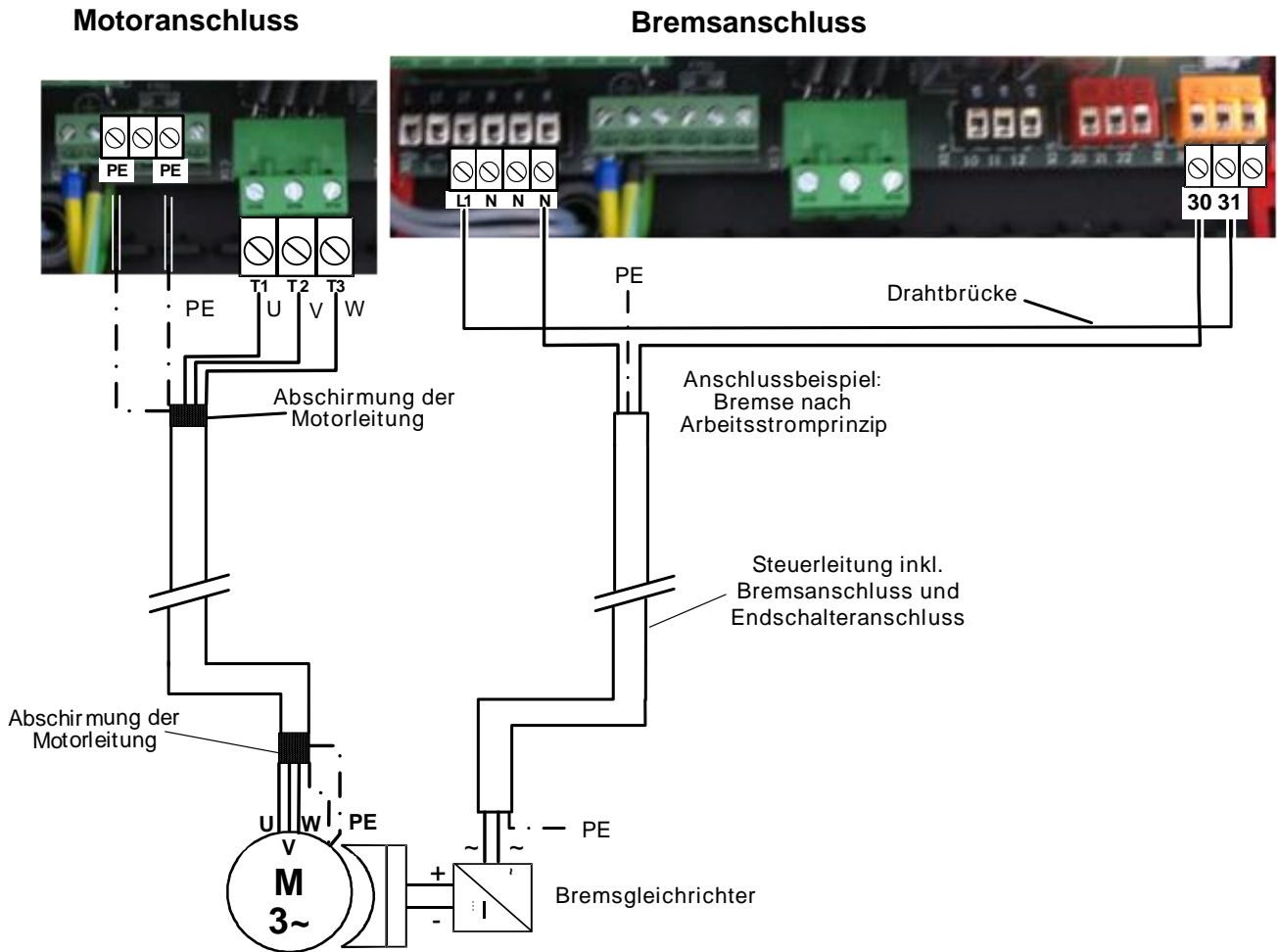
Abbildung 5: Motoranschluss
