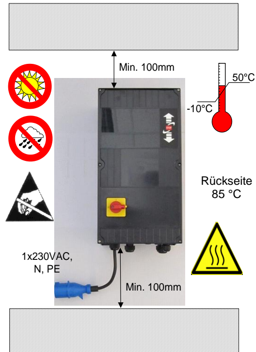
Abbildung 1: Montage der Steuerung
