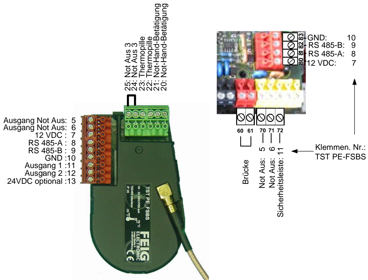
Abbildung 7: Absolutwertgeber TST PE FSB
