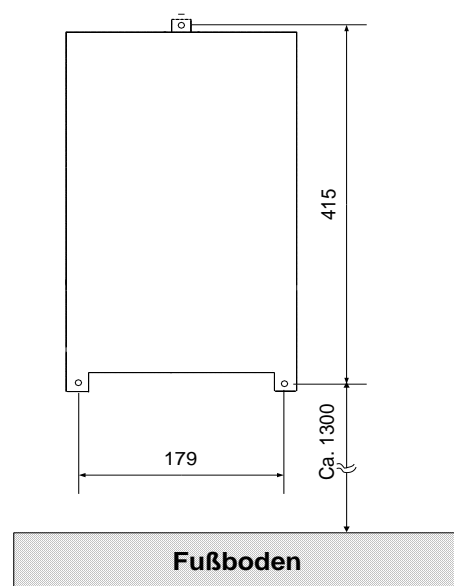
Abbildung 2: Bohrplan
