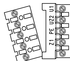
Abb. 5: Motorstecker für Wechselstrommotore mit symmetrischer Wicklung
