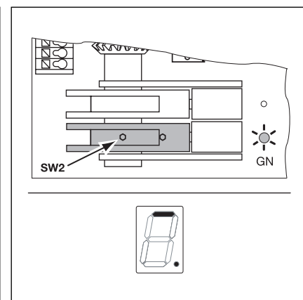
6-2.5 Nocken festsetzen, Anzeige Endlage Tor-Auf
