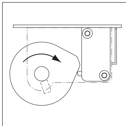
6-3.3 Schaltrichtung des Schaltnockens Tor-Zu, Montageart „Horizontal“
