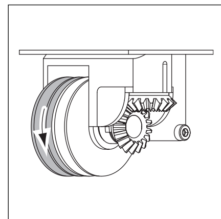
6-2.3 Drehrichtung des Schaltnockens Tor-Auf (Farbe Grün)
