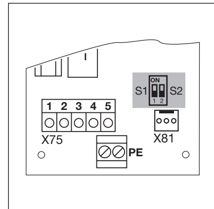
7-4.2 Betriebsarten-Wahlschalter S1/S2
