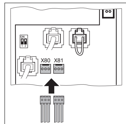
4-4.3 Anschluss der Relaisplatten an X80/X81
