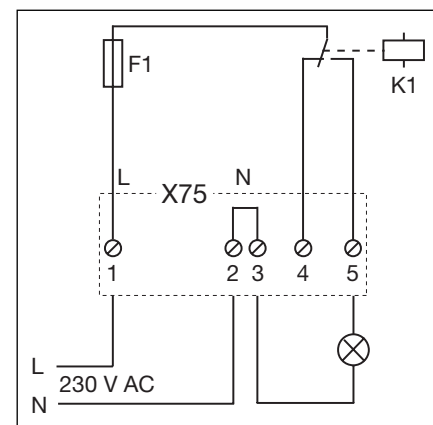
7-4.3 Schaltplan Relais und Anschlussbeispiel für 230 V Lampe
