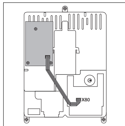
7-1.3 Montage einer Erweiterungsplatine in Breite einer Teilungseinheit im Steuerungsgehäuse und Kabelführung für X80.
